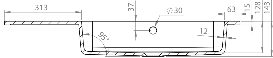
PRZEKRÓJ N-N SKALA 1 : 8
